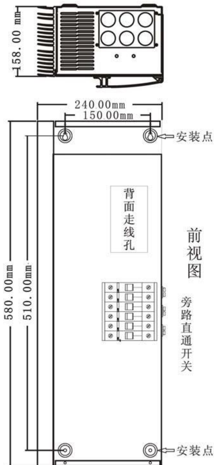
安装尺寸图
