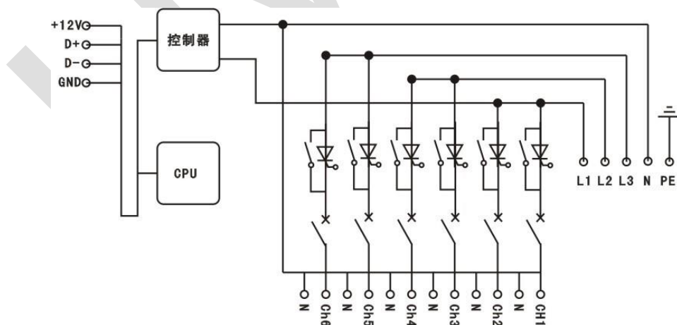
控制电路图
